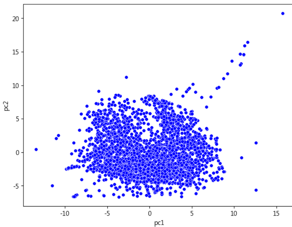
圖 3.2: 移除 PCA 極端值後的合成資料之 PCA 投影
